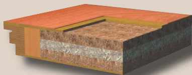
vícevrstvá konstrukce Porta (42 dB)
